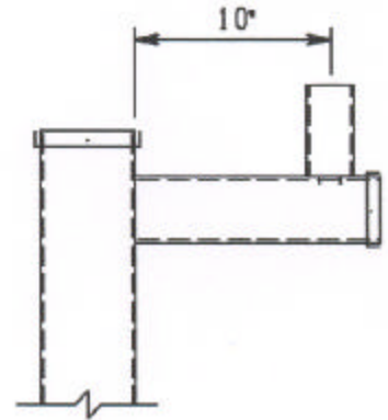
TYPE 'B'
